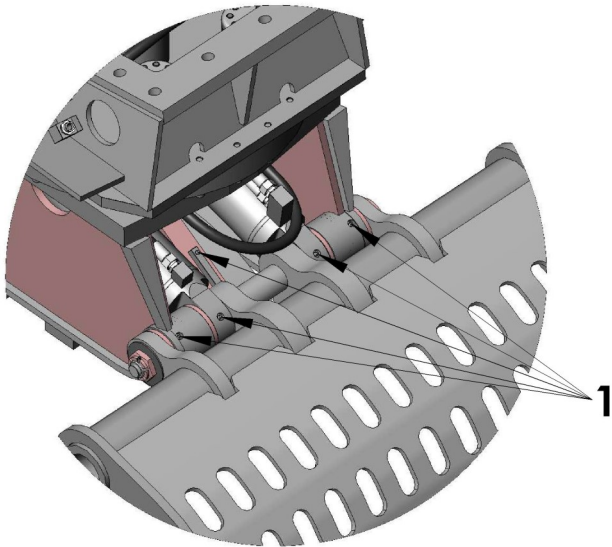
Afbeelding 3: Smering draaipunten
